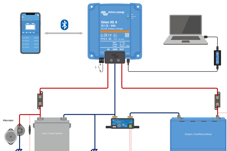
Normale impostazione del collegamento come caricabatterie CC-CC
