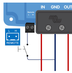
c) Cablaggio pin L
