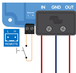
a) Cablaggio pin L-H
